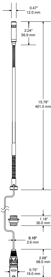
PRO 47TL Dimensions
