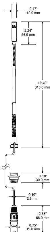
PRO 47T Dimensions
